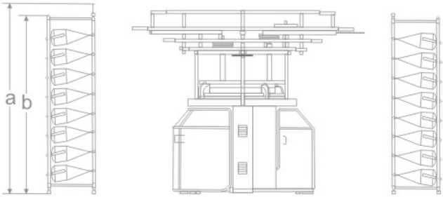
机器尺寸图 MACHINE BODYSIZE DRAWING
